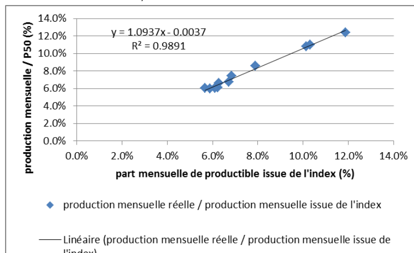
graphique 1 : productions mensuelles de la centrale et productions issues de l'index, données MERRA-2 sans correction de densité
