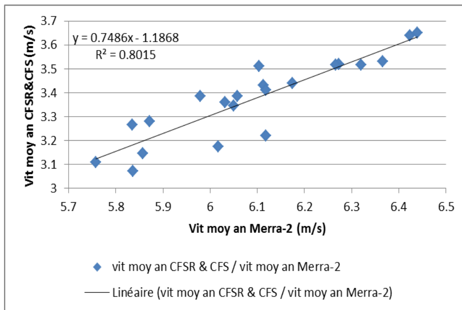
graphique 3 : corrélation entre les CFSR/CFS et les Merra-2, 1995-2015, Marne
