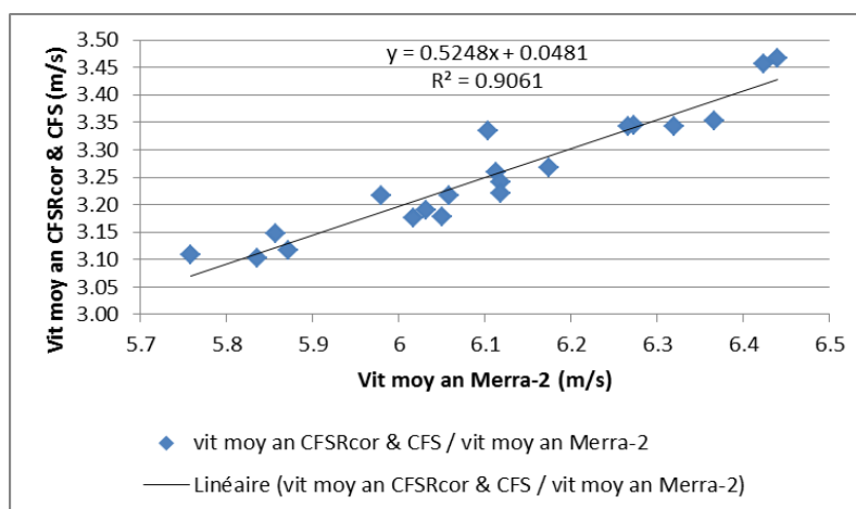
graphique 6 : corrélation entre les CFSRcor & CFS et les Merra-2, 1995-2015, Marne
