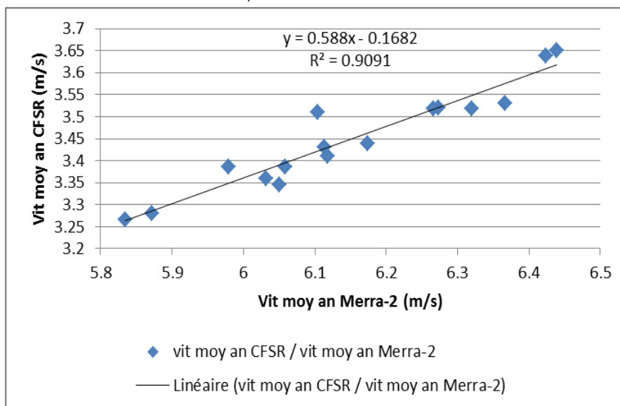
graphique 4 : corrélation entre les CFSR et les Merra-2, 1995-2010, Marne
