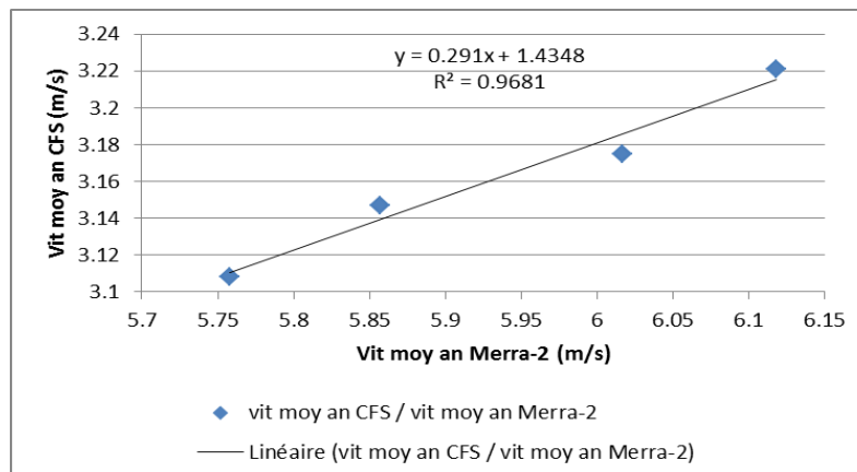
graphique 5 : corrélation entre les CFS et les Merra-2, 2012-2015, Marne
